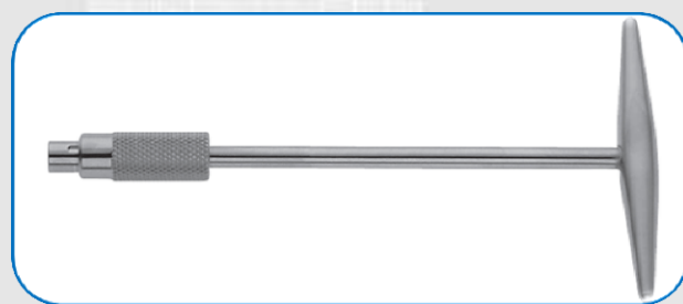
AO coupling T-handle
